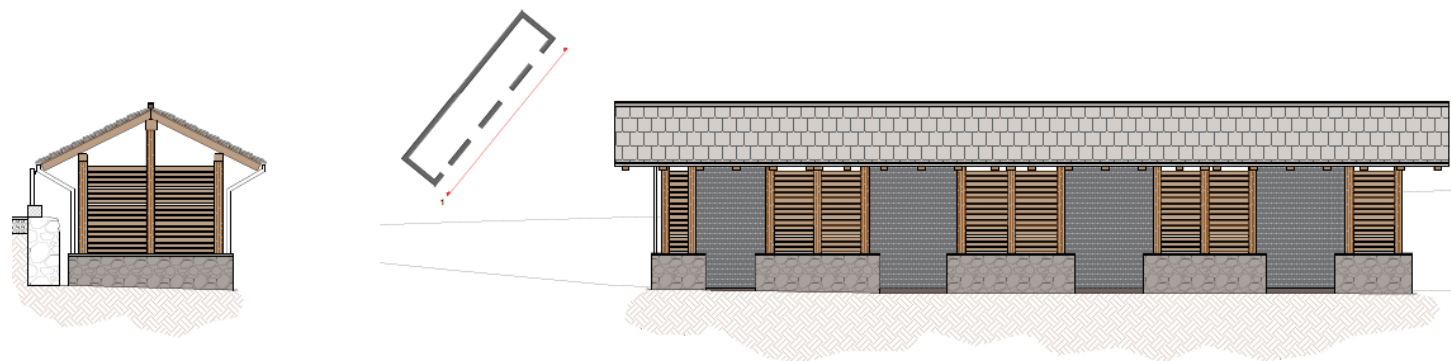
PROSPETTO 1 - Scala 1:50
