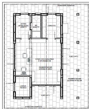
PIANTA EDIFICIO ACCOGLIENZA 1:50
